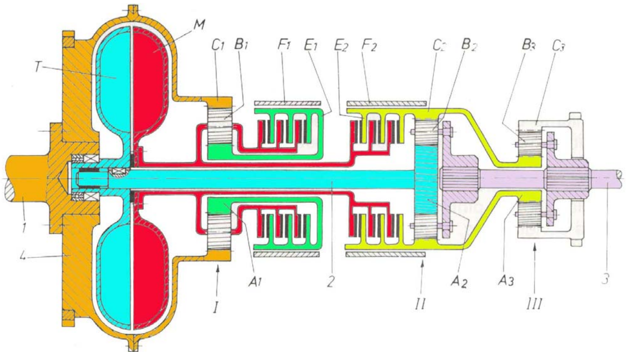
Fig. 2.11B Esquema de la caja de cambios automática (Hidra-Matic).
